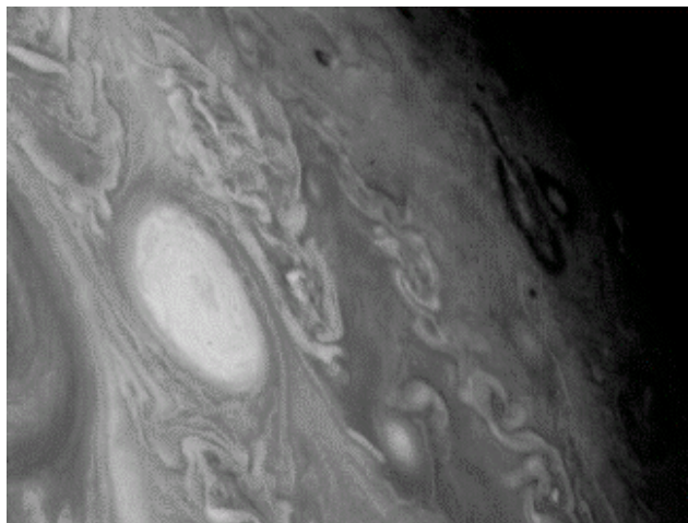
Ausschnitt aus der Jupiteratmosphäre, aufgenommen von VOYAGER 2 (NASA)
